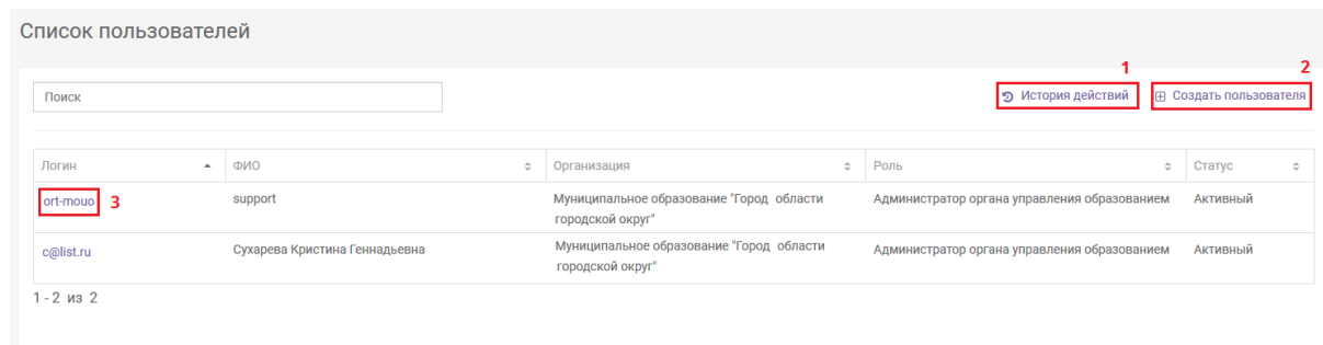
Рисунок 18 – «Панель администратора»
